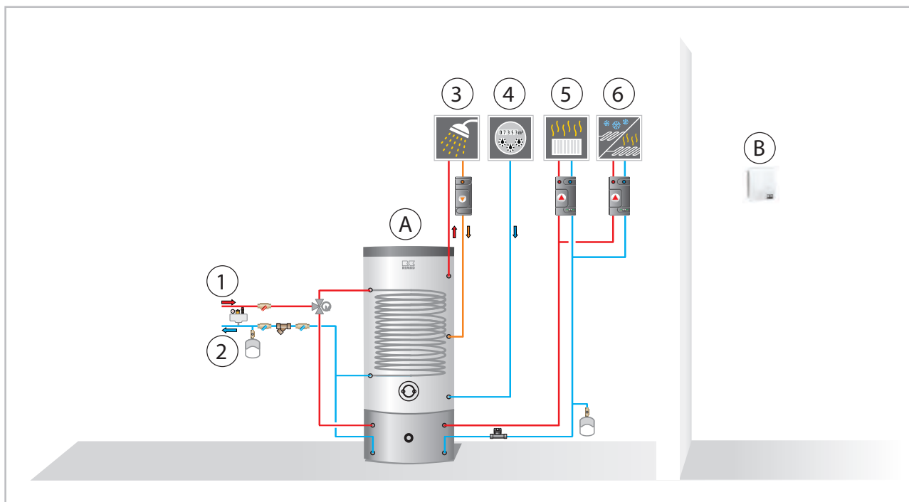
Abb. 8: Beispiel Hydraulikschema
