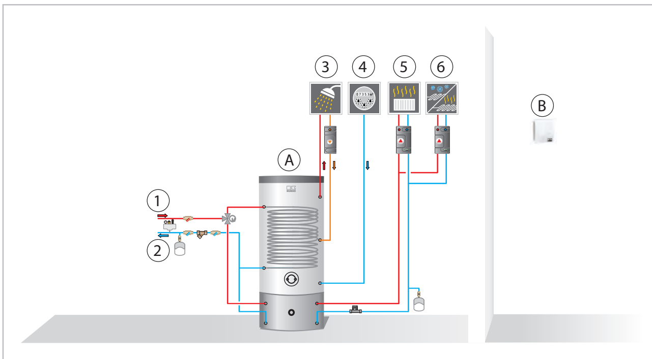
Abb. 12: Beispiel Hydraulikschema
